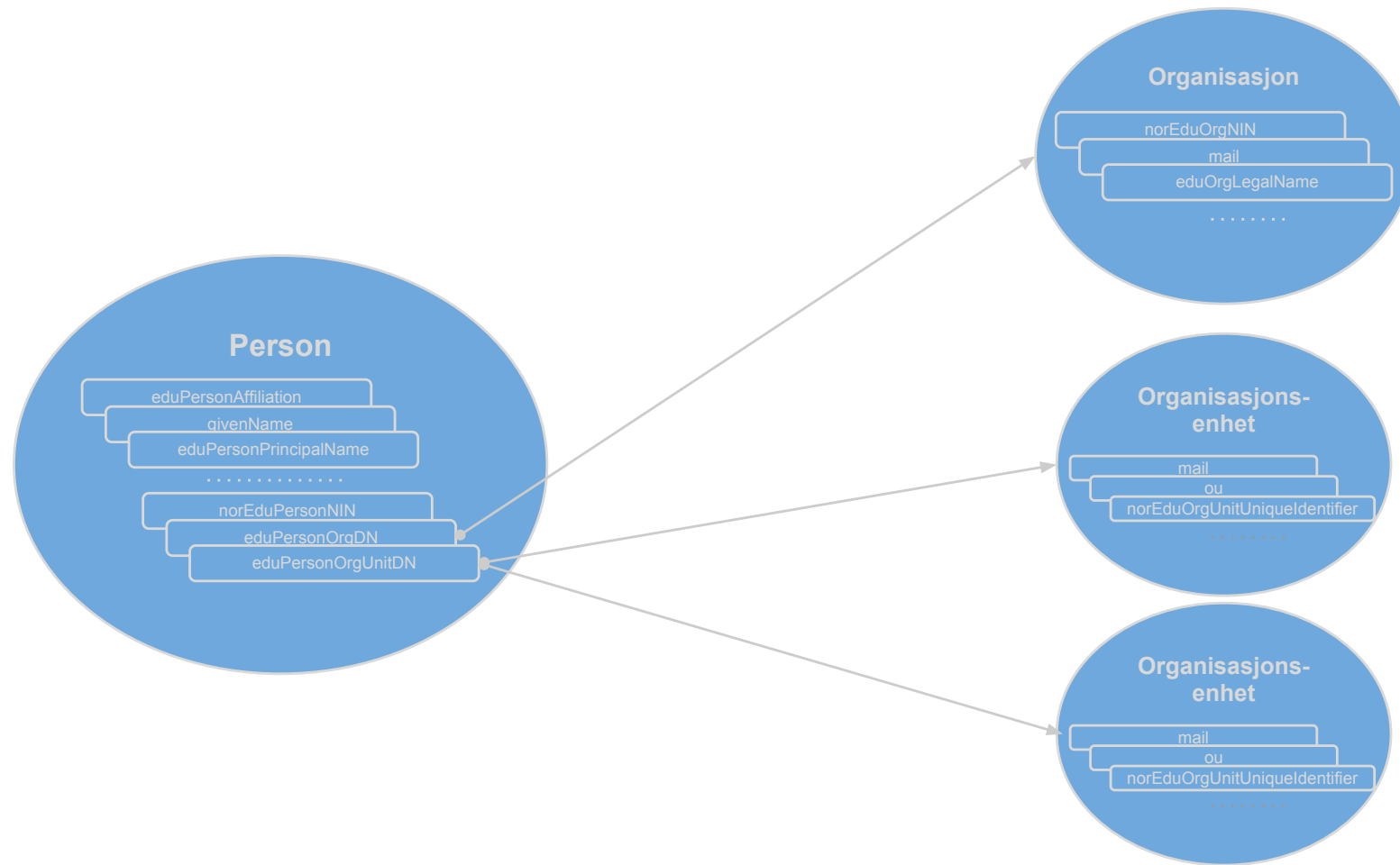
Figur 1: De ulike objektclassene i Feide-katalogen: person, organisasjon og organisasjonsenhet. Pilene viser hvordan bestemte attributter i person-noden peker på den organisasjon og organisasjonsenhet(er) personen tilhører.
